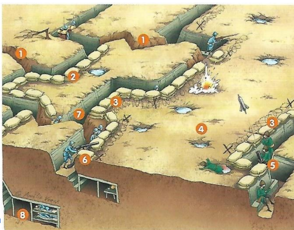
Schéma d'une zone de front
